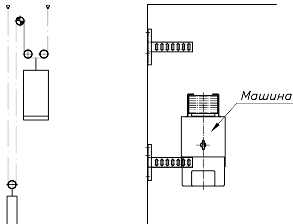
Кинематична схема на носещите въжета/ремъци
