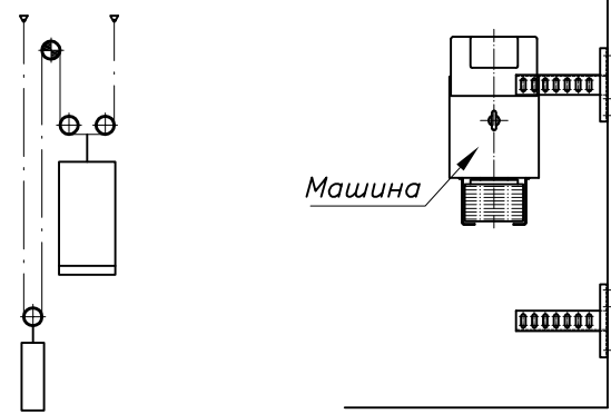
Кинематична схема на носещите възжета/ремъци
